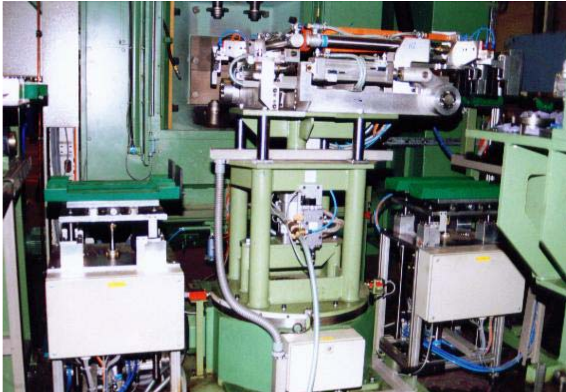
Abb. 1: Handlingsystem zum Bestücken eines Strahlofens mit Achsfedern
